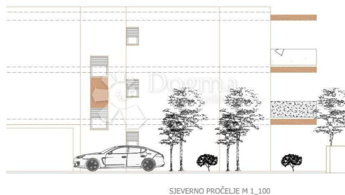
SJEVERNO PROČELJE M 1_100
