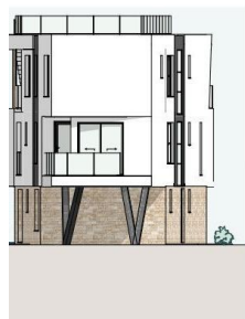
CELJE 1:100
