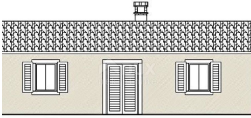
SJEVEROZAPADNO PROČELJE
